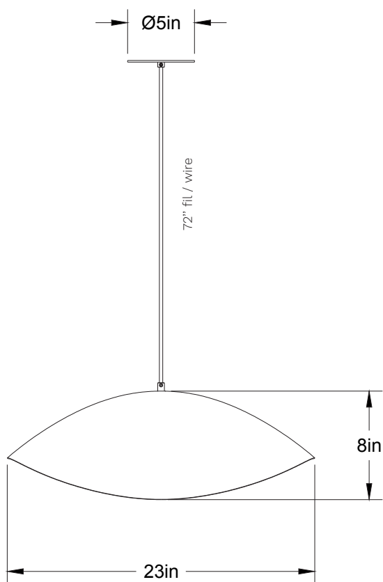
Avant/Front
